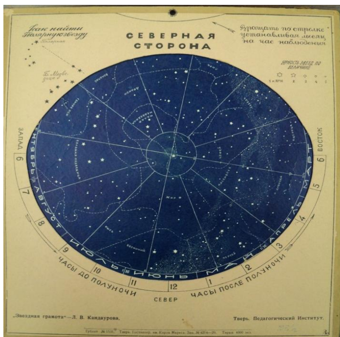
Звездная грамота. Подвижная карта звездного неба (северная сторона)
