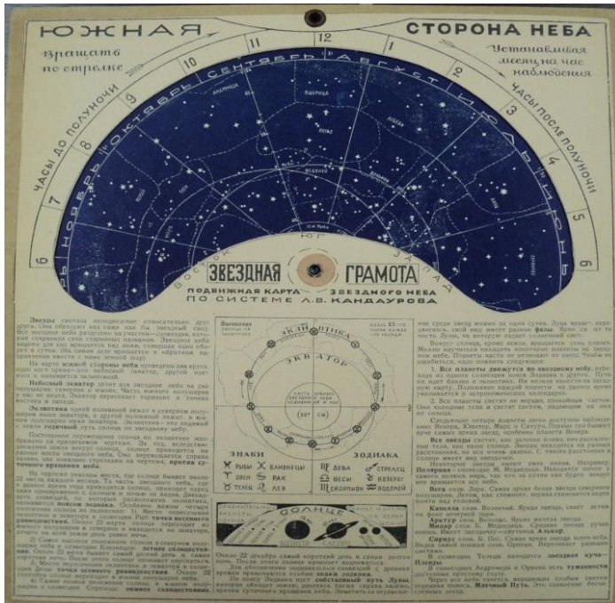
Звездная грамота. Подвижная карта звездного неба (южная сторона)
