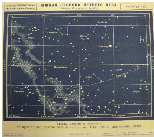
Сезонные карты звездного неба
