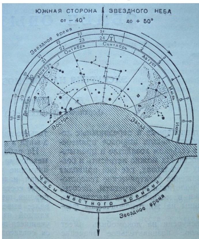
Звездная карта с заслонкой из картона, закрывающей невидимую часть около южного полюса мира
