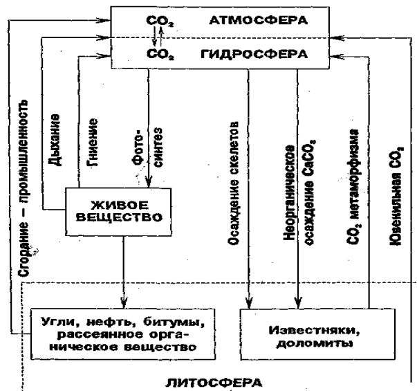
Рис.13 Круговорот углерода в биосфере Земли
