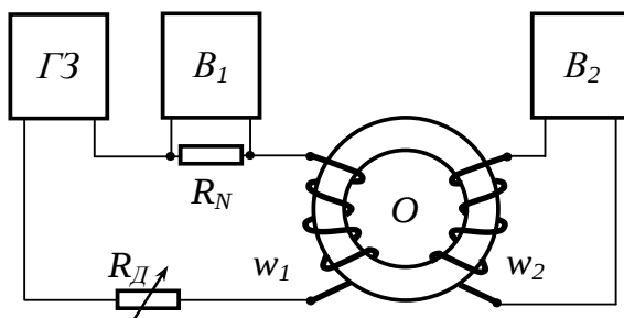
Рис. 1. ГЗ - генератор звуковых сигналов; B_1 и B_2 - вольтметры переменного тока; O - образец; w_1 и w_2 - намагничивающая и измерительная обмотки; R_N – одноо́мное сопротивление; R_{\text{Д}} – добавочное сопротивление
