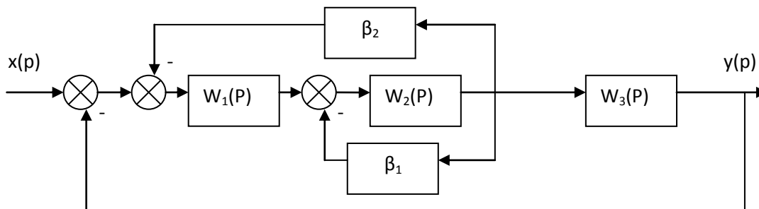
Вариант структурной схемы по условию задачи № 2
