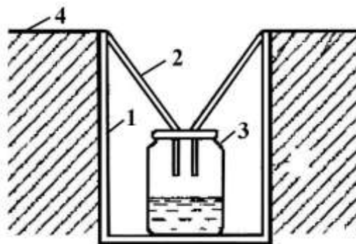
Рис. 7. Ловушка с воронкой: 1 – наружный цилиндр; 2 – воронка; 3 – банка с фиксирующей жидкостью; 4 – дно канавки (по Тихомировой, 1975)
