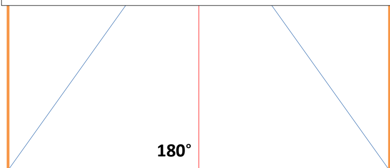
Рис. 1. Система разграфки листа формата А4 для создания картографической сетки полярной азимутальной проекции
