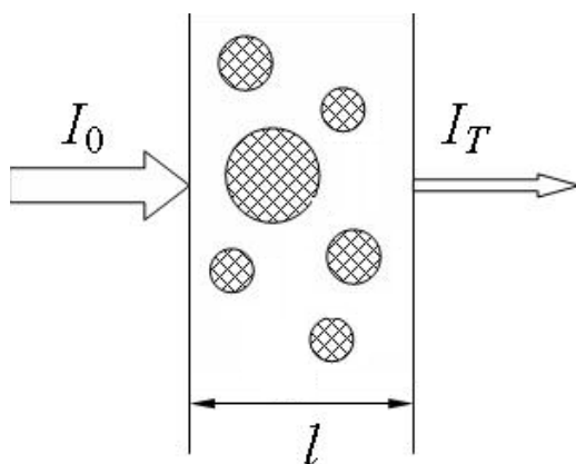
Рис. 1. Схема взаимодействия электромагнитного излучения с веществом
