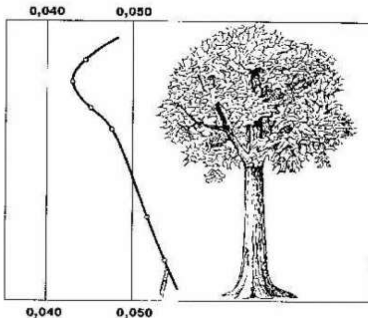
Рисунок 1. Кривая, показывающая изменения содержания \text{CO}_2 (%) в различных слоях воздуха вблизи дерева
